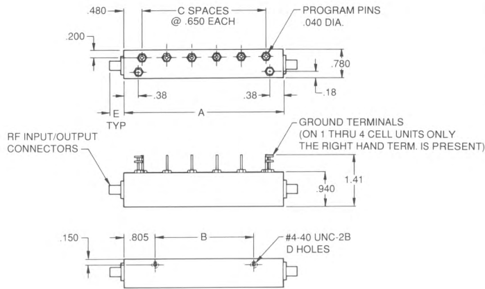
OUTLINE 1A
